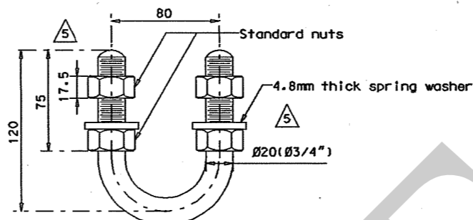
M20 U-BOLT
