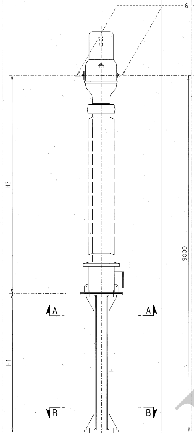
ELEVATION
