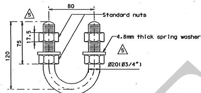
M20 U-BOLT
